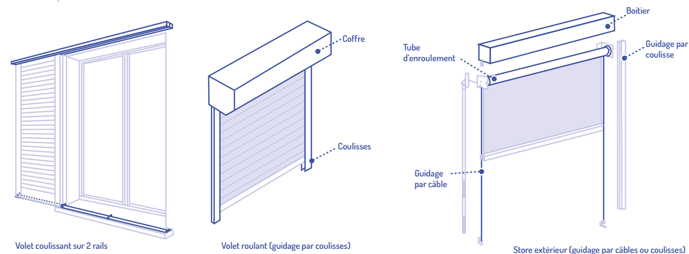
Exemples de systèmes de guidage
